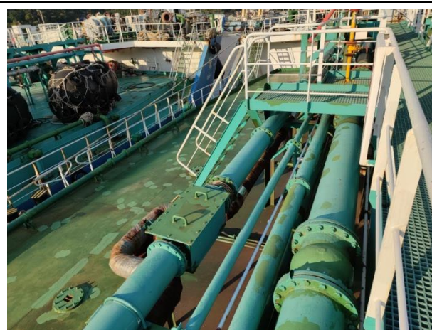
甲板导热油管路
